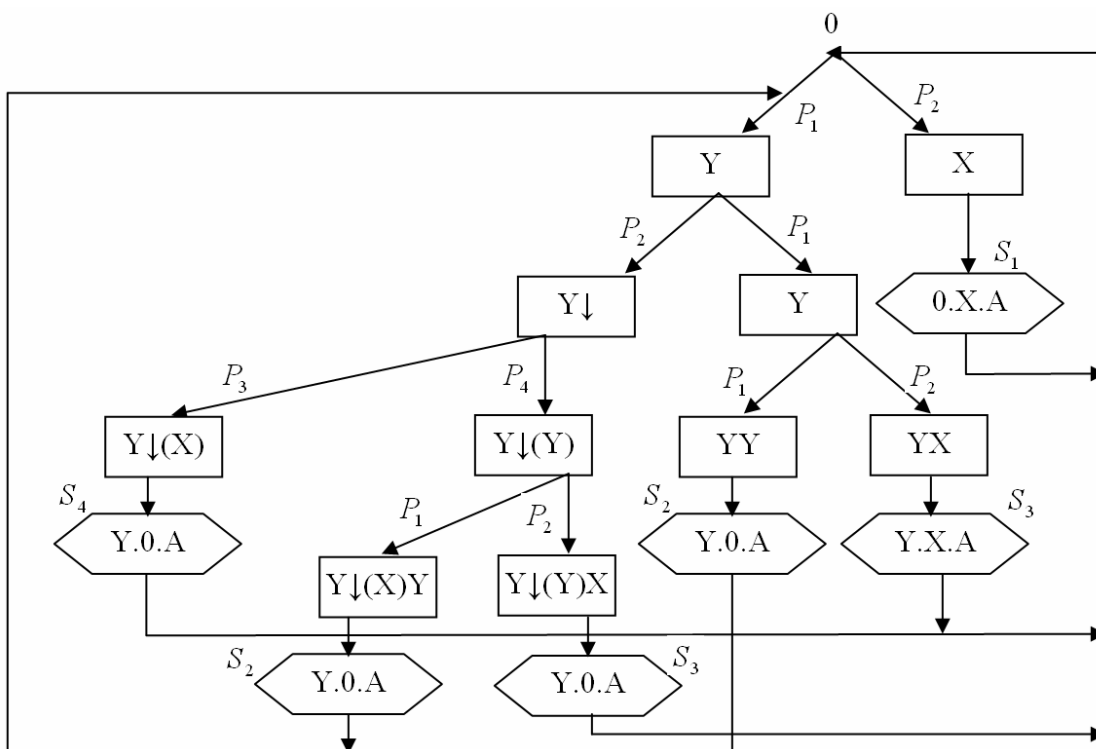
Рисунок 6 – Процес породження мікрокоманд (H, G) = (1, 1)
