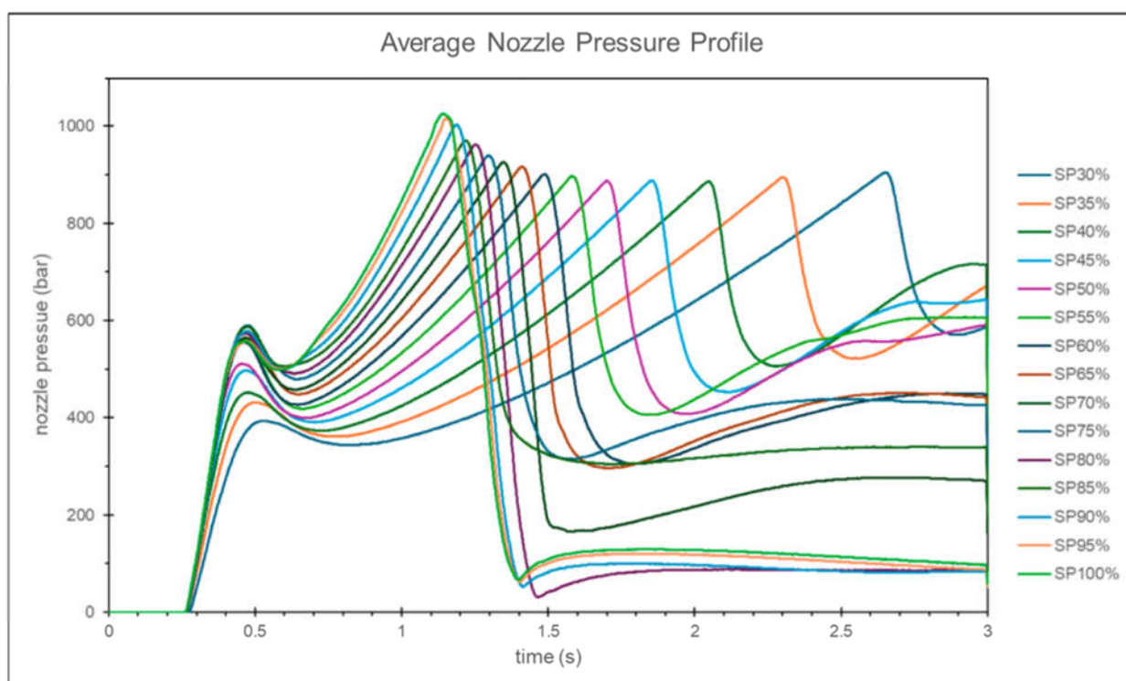
Рисунок 2 – Експериментальні криві тиску в соплі при різних швидкостях впорскування [3]
