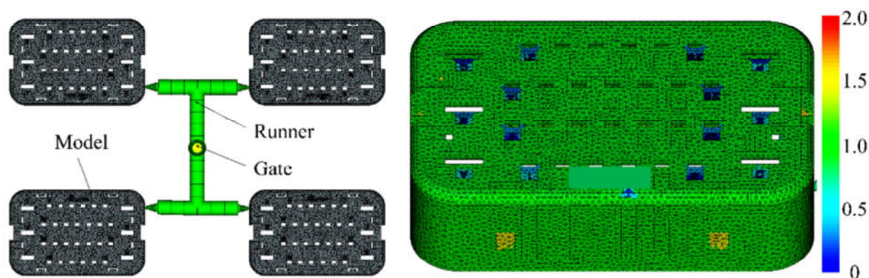
Рисунок 1 – Сітка моделі в «Autodesk Moldflow» [1]
