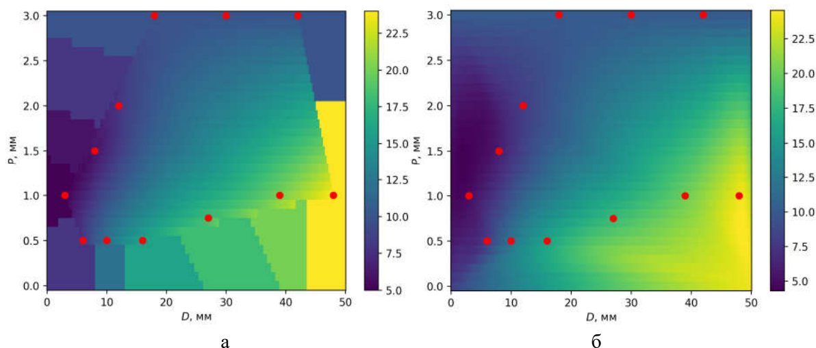
Рисунок 4 – Інтерпольовані залежності швидкості різання машинними мітчиками зі сталі Р6М5 ( V , м/хв) в заготовках з конструкційної сталі від діаметра ( D ) і кроку ( P ) різби: поєднання CloughTocher2DInterpolator та NearestNDInterpolator (а); використання додаткових кутових точок та CloughTocher2DInterpolator (б)
