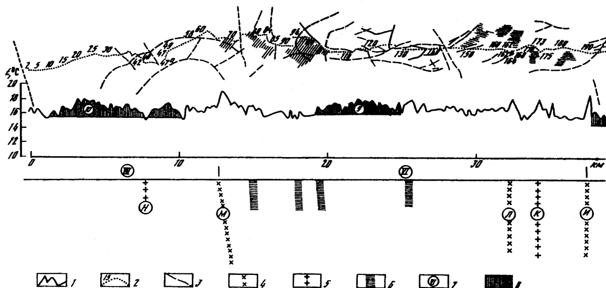
1 – температура на глибині 1,5 м (°С); 2 – профіль з пікетами; тектонічні порушення: 3 – в осадовому чохла, 4 – глибинні; 5 – встановлені за результатами геотермічних досліджень, 6 – зони дроблення; 7 – блоки різної геотермічної активності; 8 – локальні структури
