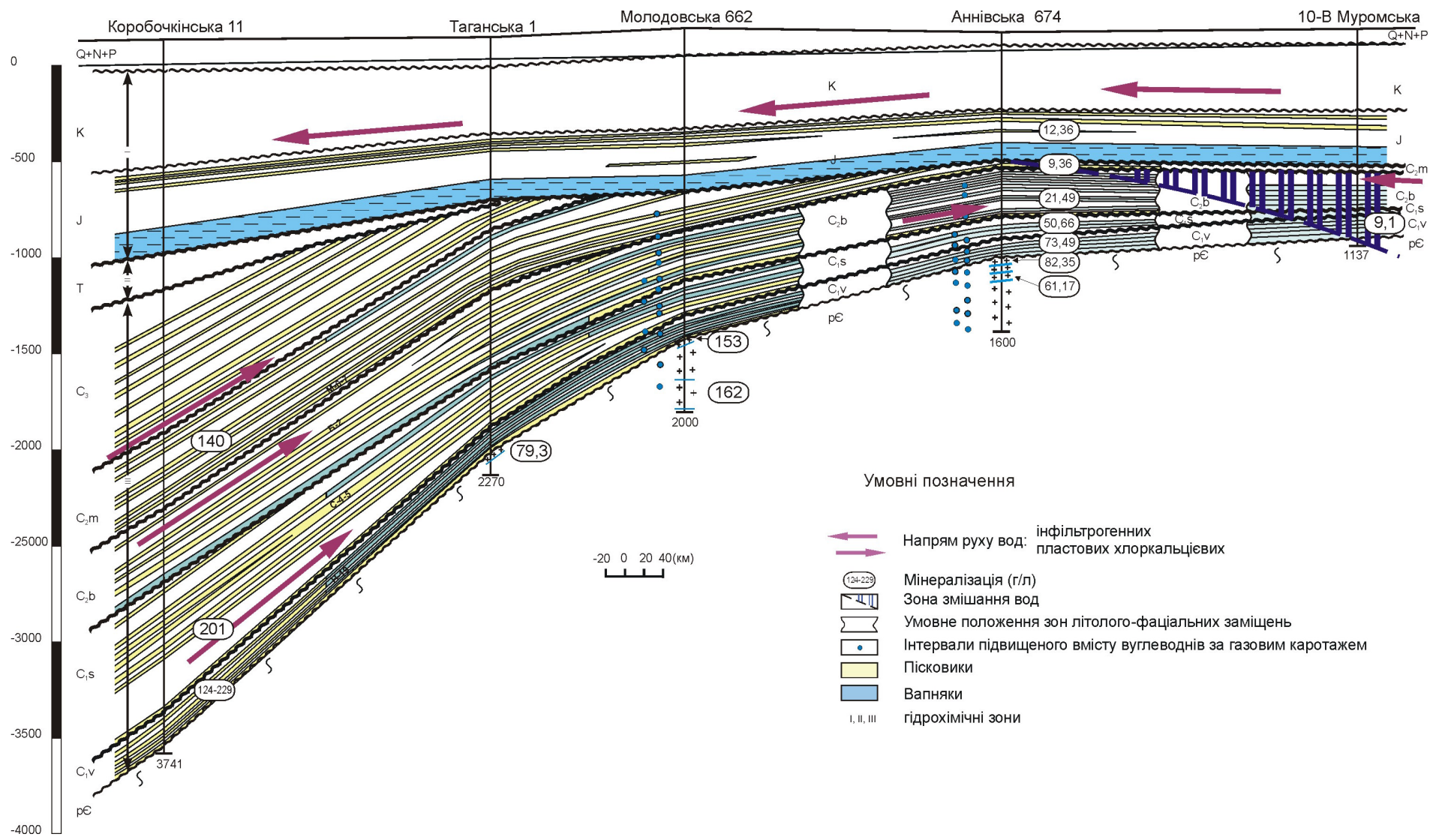
Рисунок 3 — Профільний гідрогеологічний розріз північного борту ДДЗ (за І.В.Височанським, 1999)
