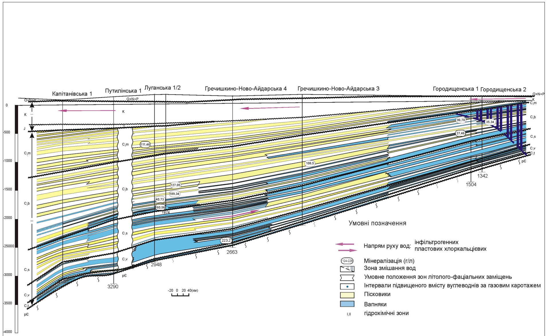
Рисунок 4 — Профільний гідрогеологічний розріз північного борту ДЗ
