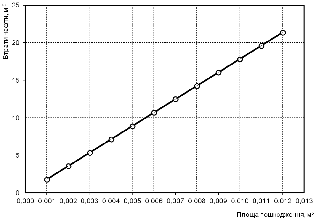
Рисунок 4 – Графічна залежність аварійних втрат нафти від площі пошкодження нафтопроводу для розрахункової схеми 2
