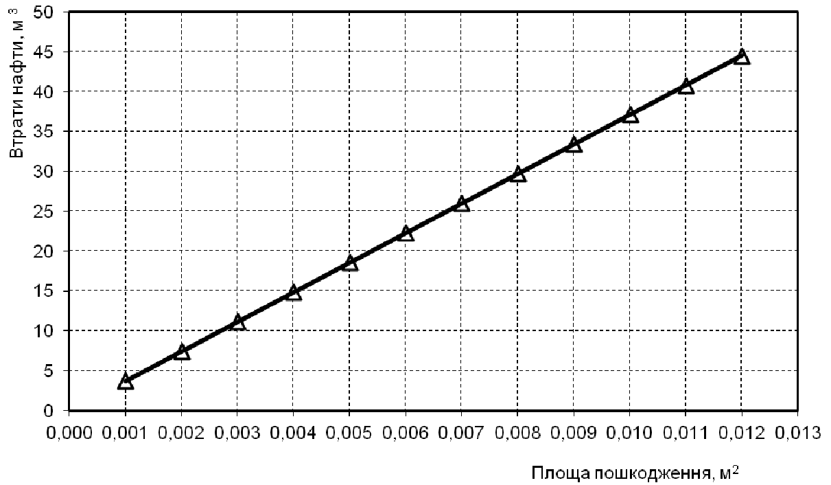
Рисунок 3 – Графічна залежність аварійних втрат нафти від площі пошкодження нафтопроводу для розрахункової схеми 1
