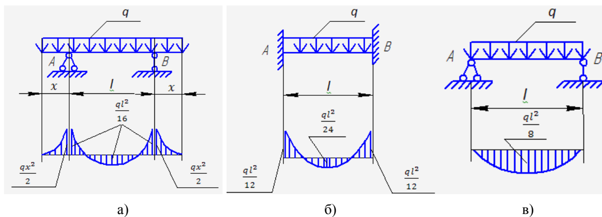
Рисунок 1 – Схеми балкових переходів
