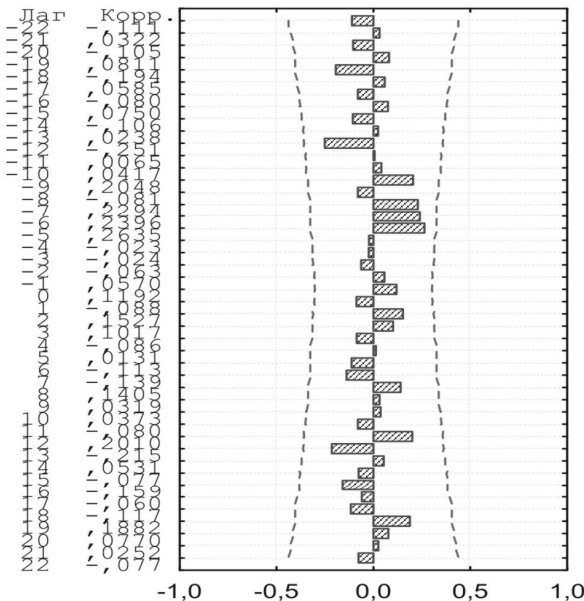
Функція взаємної кореляції активізації зсувів та сумарної енергії землетрусів ( L_n )
