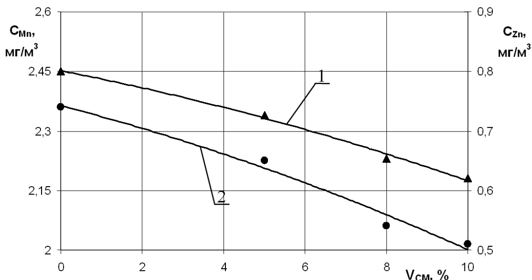
Рисунок 2 – Залежність концентрації C_{Zn} , C_{Mn} у відхідних газах двигуна ЗІЛ-130 від відсоткового об'ємного вмісту у паливі SM , V_{SM}
