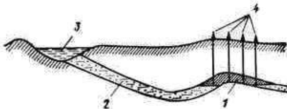
Рисунок 1 – Схема геологічних умов існування природного водонапірного режиму
