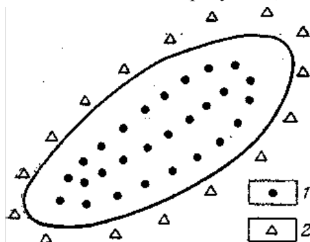
1 - видобувні свердловини; 2 - нагнітальні свердловини
