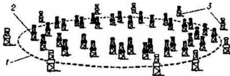
1 – контур нафтоносності; 2 – експлуатаційні свердловини; 3 – нагнітальні законтурні свердловини
