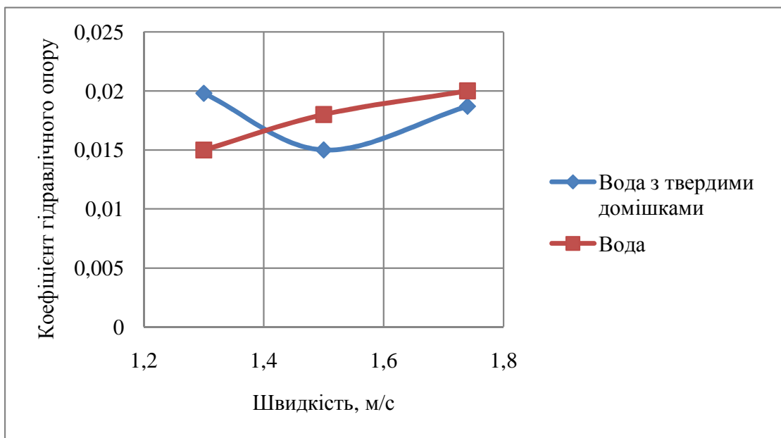
Рисунок 6 – Залежність коефіцієнта гідравлічного опору від швидкості за концентрації гумової крихти c = 0,5 \%
