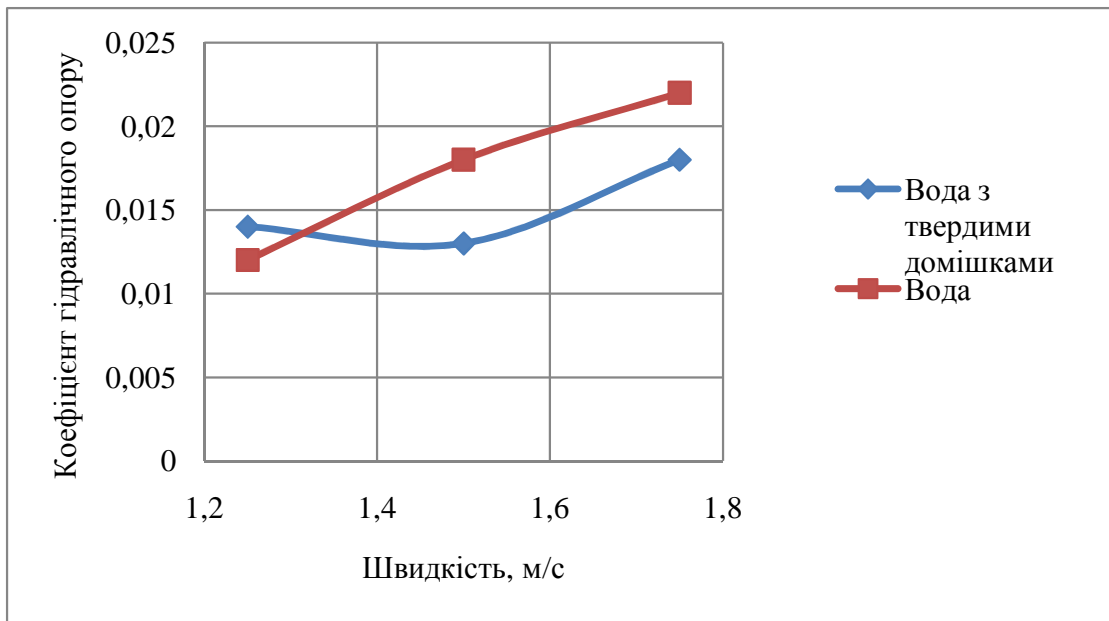
Рисунок 5 – Залежність коефіцієнта гідравлічного опору від швидкості за концентрації гумової крихти c = 0,25 \%
