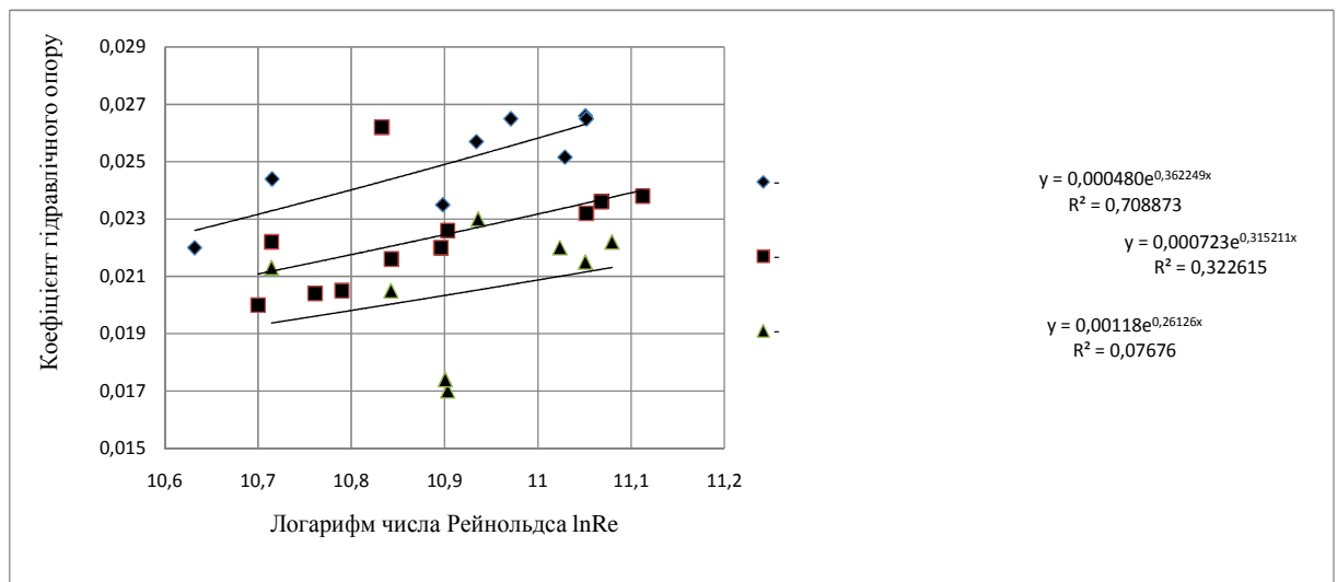
Рисунок 3 – Залежність коефіцієнта гідравлічного опору від числа Рейнольдса за концентрації твердих домішок c = 1\% .
