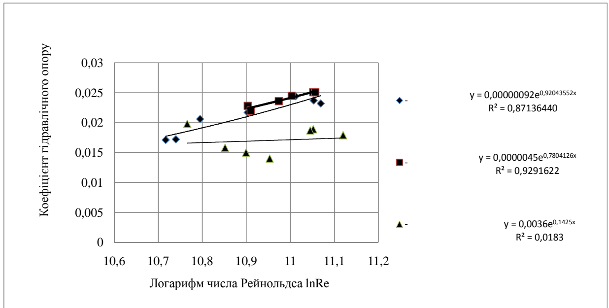
Рисунок 2 – Залежність коефіцієнта гідравлічного опору від числа Рейнольдса за концентрації твердих домішок c = 0,5\%
