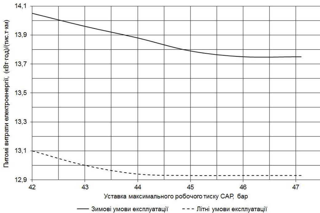
Рисунок 2 – Динаміка зміни питомих витрат електроенергії на перекачування нафти від величини уставки максимального робочого тиску САР за схеми роботи насосних агрегатів 1п,1,2-1-2,3-2
