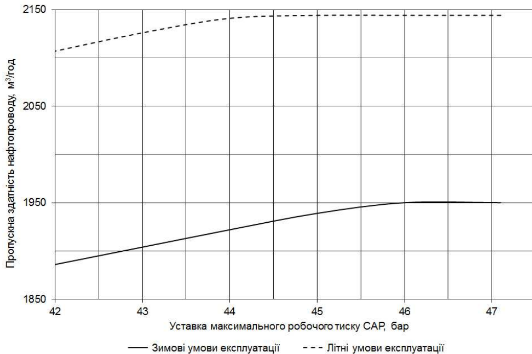
Рисунок 1 – Динаміка зміни пропускної здатності магістрального нафтопроводу від величини уставки максимального робочого тиску САР за схеми роботи насосних агрегатів 1п,1,2-1-2,3-2
