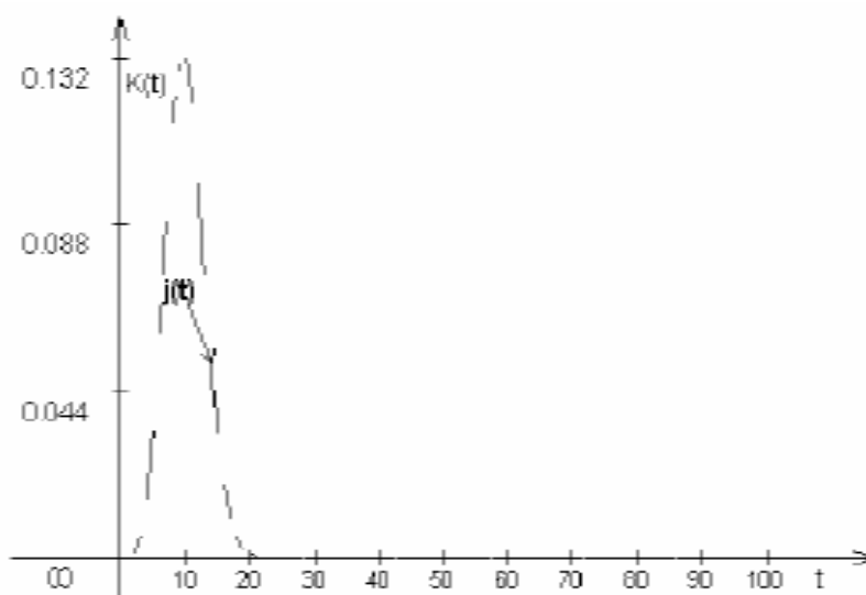
Рисунок 2 – Функція стрибків при n=0, 1, 2, 3, 4 ; T=100 ; \rho=0,1
