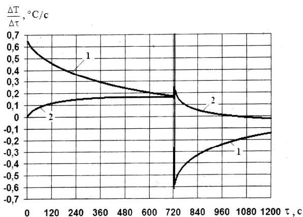
Рисунок 2 – Темпи нагрівання обода 1 і бічної стінки 2 заднього гальмівного барабана автотransпортного засобу ЗІЛ-130 в перебігу випробувань типу II та при вимушеному охолодженні тривалістю 480с
