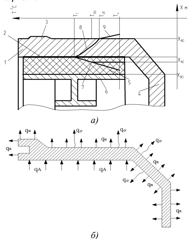
1 - гальмівний барабан; 2, 3, 4 - обід, що має підкріплююче кільце і бічна стінка барабана; 5 - фрикційна накладка; 6 - гальмівна колодка; 7, 8, 9 - криві зміни температури по товщині накладки, обода і в повітрі, що омиває його зовнішню поверхню
