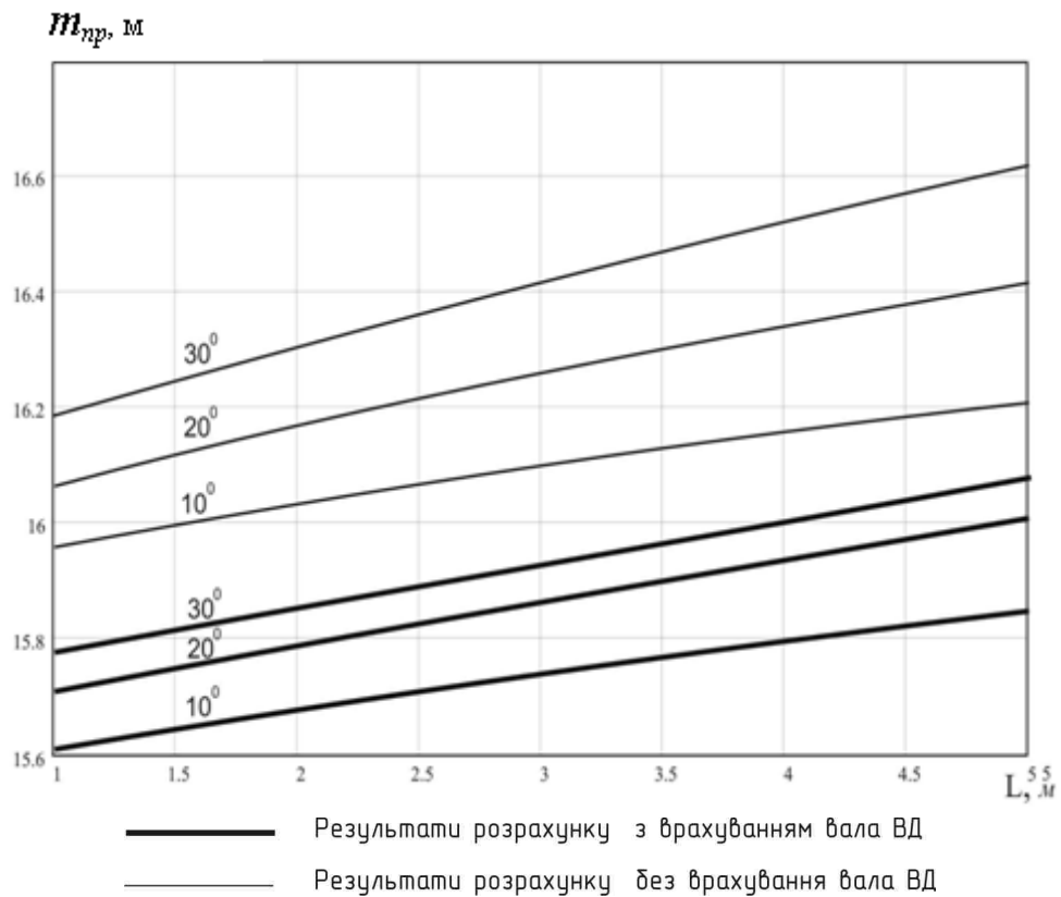
Рисунок 9 – Залежність зміни приведенного значення однієї безрозмірної одиниці довжини t_{пр} КНБК від відстані між ОЦЕ і долотом
