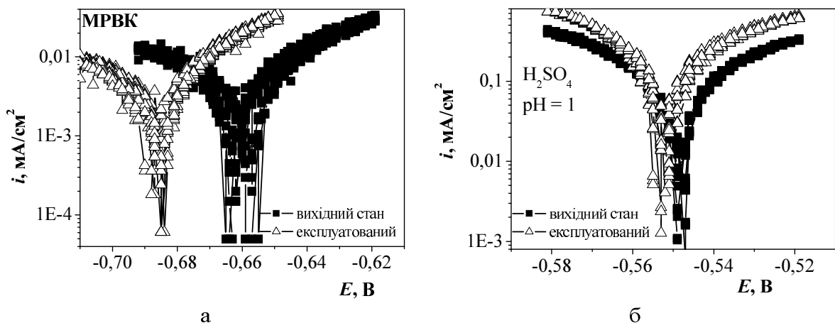
Рисунок 6 – Поляризаційні криві сталі 10Г2С, зняті у модельному розчині водного конденсату у газовій трубі (а), та у розчині H 2 SO 4 з рН=1 (б)
