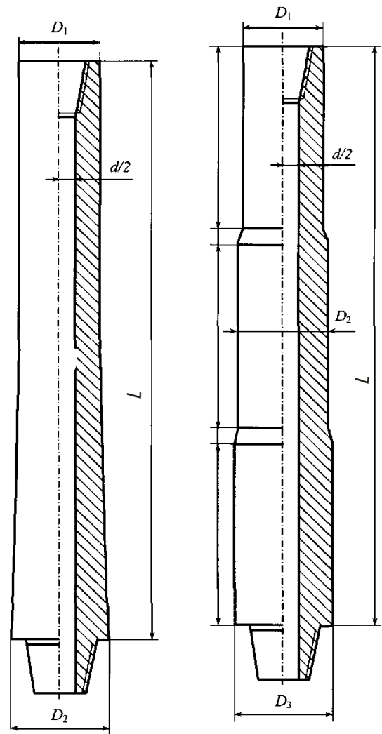
а) одноступінчаста конструкція експоненціальної форми; б) тріступінчаста конструкція
