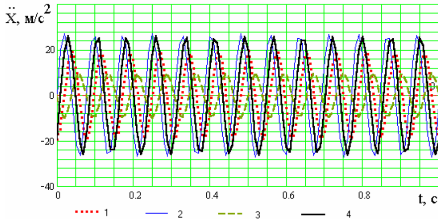
Рисунок 2 — Графіки за частоти вихідного сигналу датчика 6 Гц (а), 7 Гц (б), 10 Гц (в) і 13 Гц (г) відповідно
