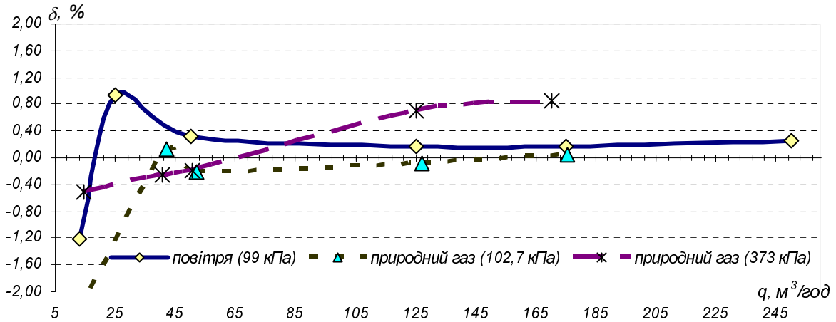
Рисунок 1 — Результати досліджень турбінного лічильника газу ЛГ-80
