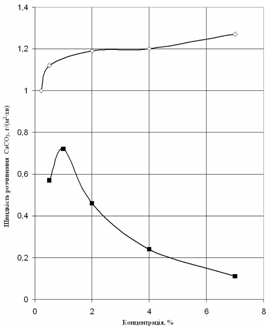
Рисунок 2 – Залежність швидкості розчинення CaCO 3 (крейди) від концентрації НТФК при температурах 80 і 95°C
