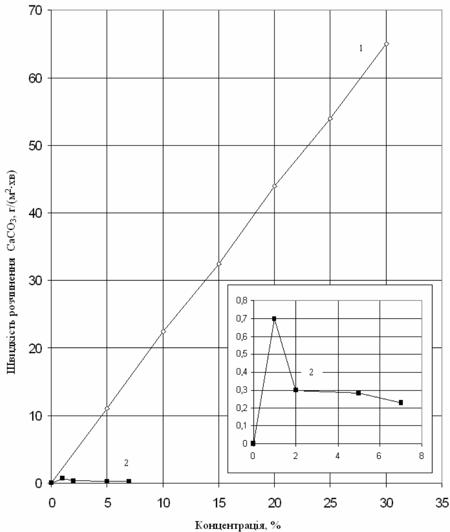
Рисунок 1 — Залежність швидкості розчинення CaCO 3 (крейди) від концентрації кислоти при температурі 60°C
