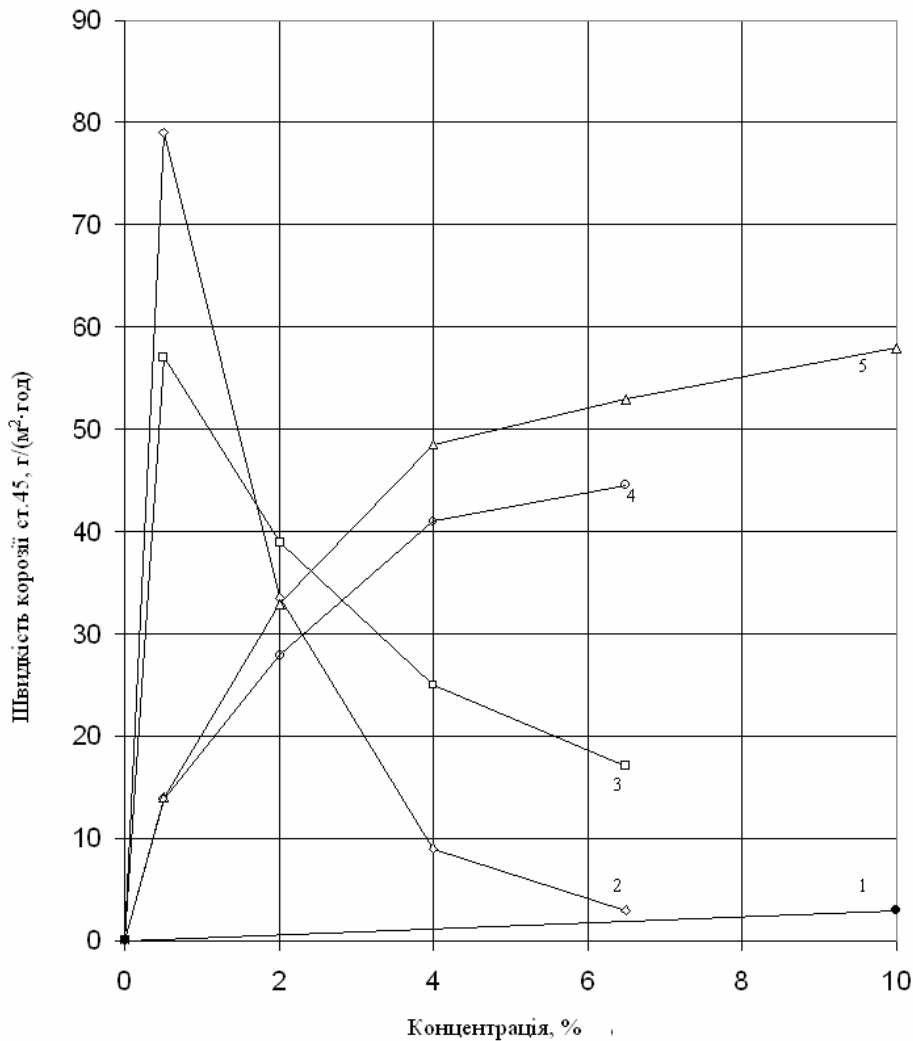
1 – HCl з додатком 0,1% КІ-1 при 60°C; 2 – НТФК при 95°C; 3 – НТФК при 80°C; 4 – НТФК при 60°C; 5 – HCl при 60°C
