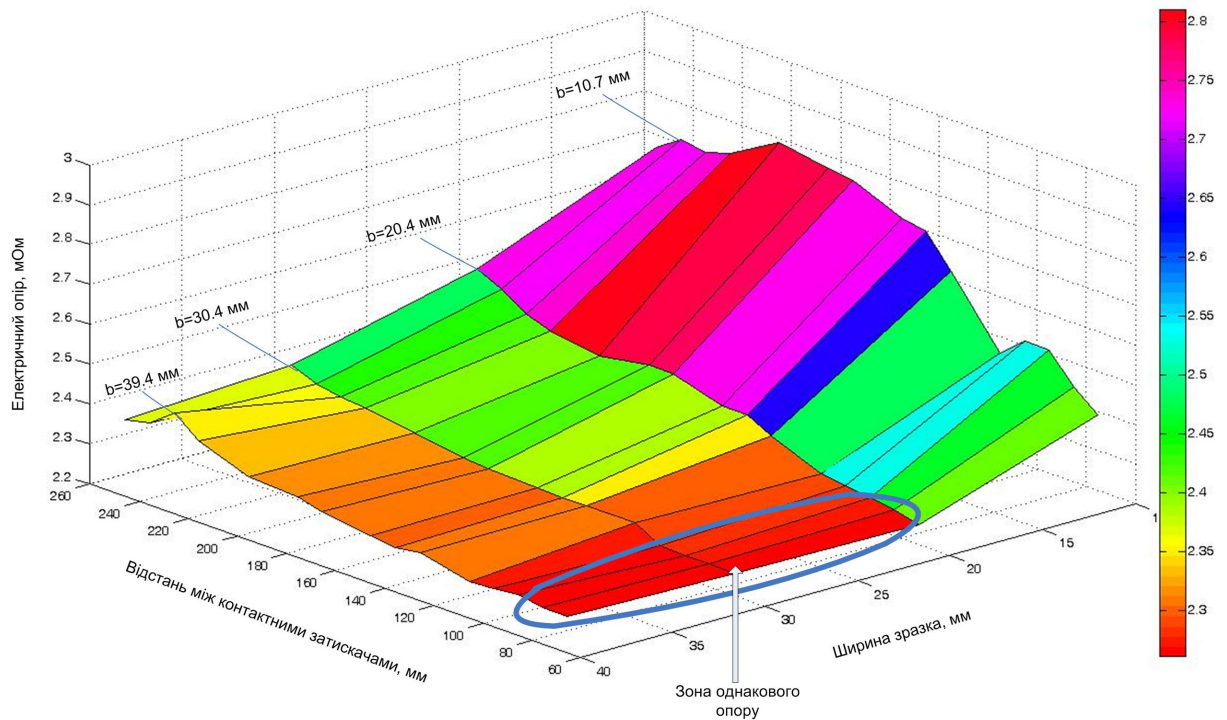
Рисунок 5 – Тривимірна поверхня залежності електричного опору від відстані між контактними затискачами і ширини сталевих зразків
