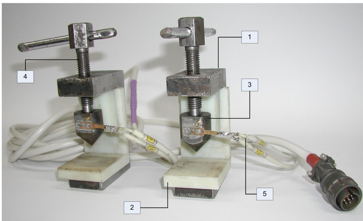
1 – струпиця; 2 – діелектрична підставка; 3 – гартований сталевий контактний наконечник; 4 – затискний гвинт; 5 – струмовий та потенціалний провідники
