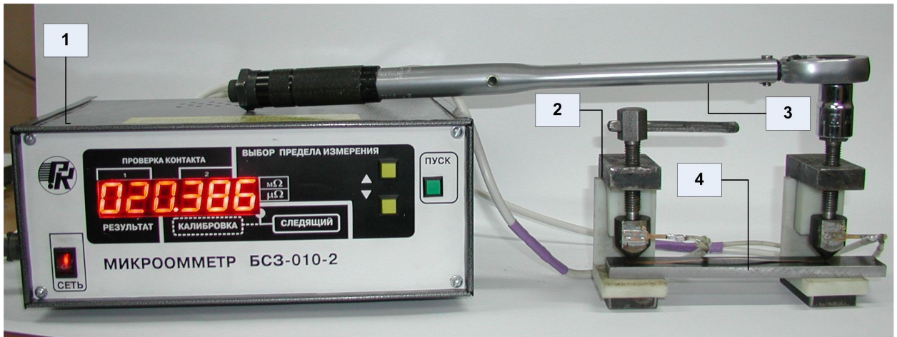
1 – мікроомметр БСЗ-010-2; 2 – контактні затискачі; 3 – динамометричний ключ; 4 – закріплений сталевий зразок
