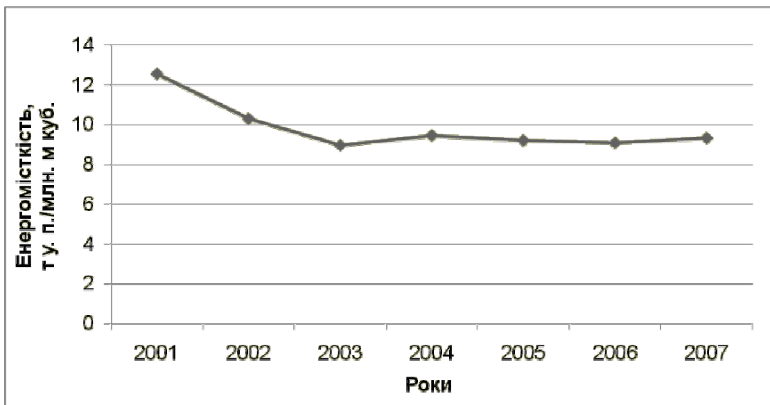
Рисунок 3 - Динаміка показника енергомiсткостi транспортування природного газу в УМГ "Прикарпаттрансгаз"
